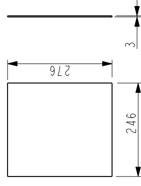
vitre x2
